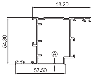
CÁNH CỬA ĐI MỞ TRONG
