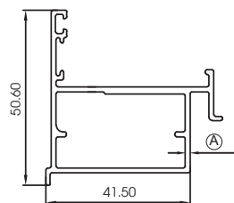
THANH ĐẢO CHIỀU
