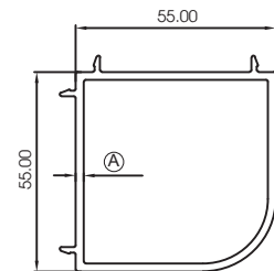
NỘI GÓC VUÔNG
