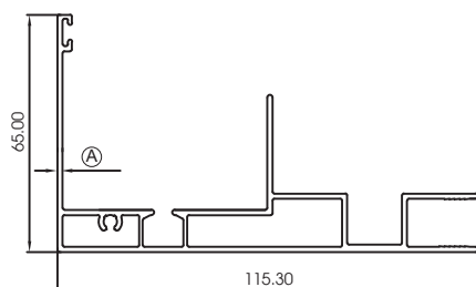
NGANG TRÊN CỬA LÙA 2 CÁCH, 4 CÁCH
