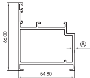
KHUNG BAO CỬA ĐI MỞ QUAY
